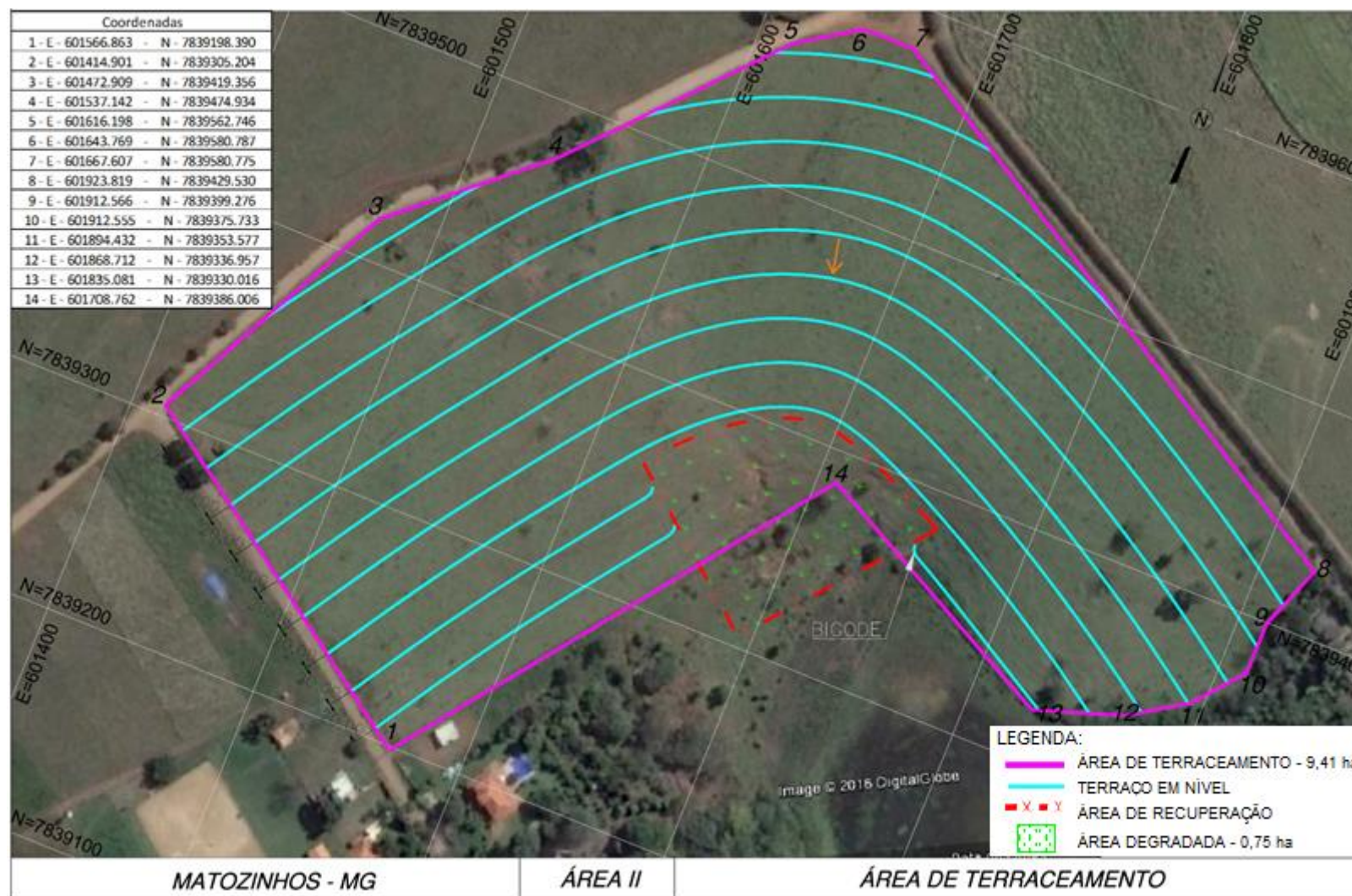
Figura 6.7 - Projeto de terraceamento da área II
