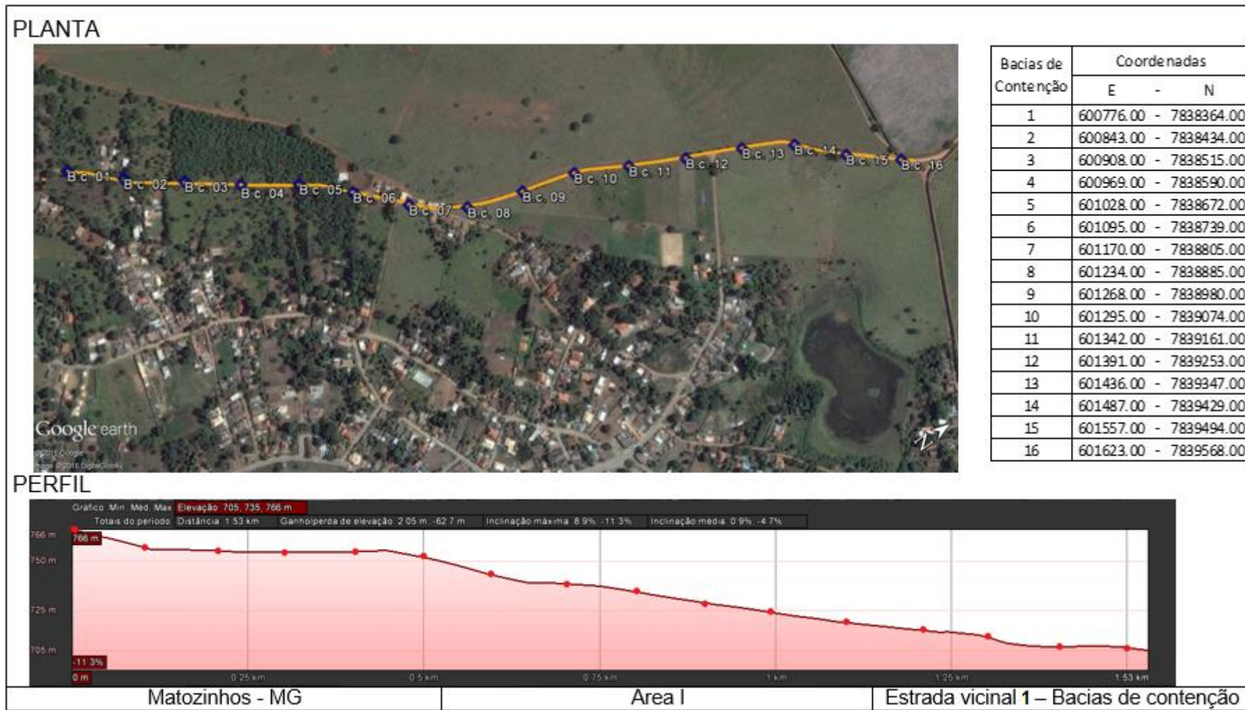
Figura 6.3– Projeto de intervenção na estrada vicinal 1, próxima à Lagoa do Fluminense
