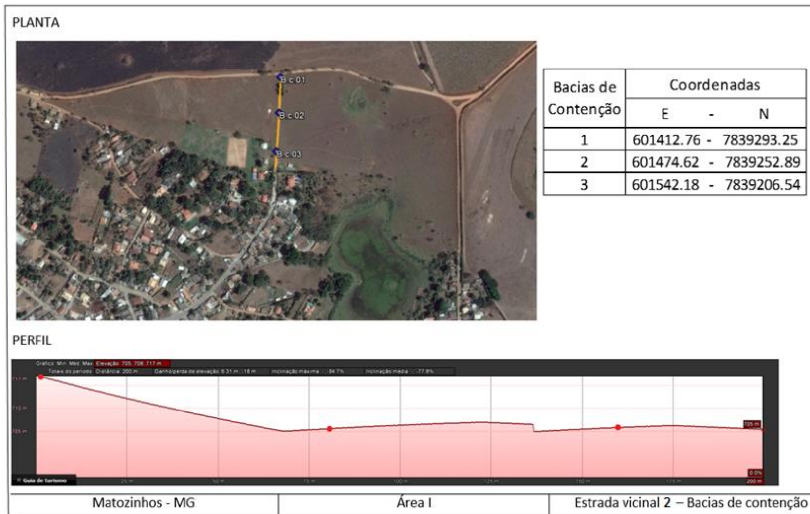
Figura 6.4 - Projeto de intervenção na estrada vicinal 2, próxima à Lagoa do Fluminense
