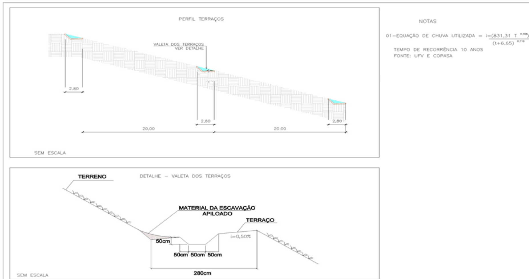
Figura 6.8 - Perfil dos terraços
