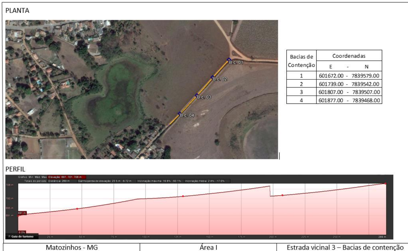
Figura 6.5 - Projeto de intervenção na estrada vicinal 3, próxima à Lagoa do Fluminense
